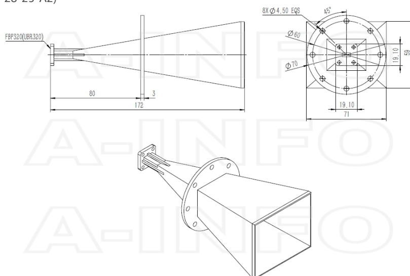
FBP320 Output (P/N: LB-28-25-A2)
